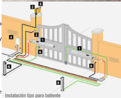
Instalación tipo para batiente
